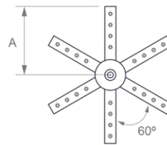
Vista Superior Mod. PDC 6.4
